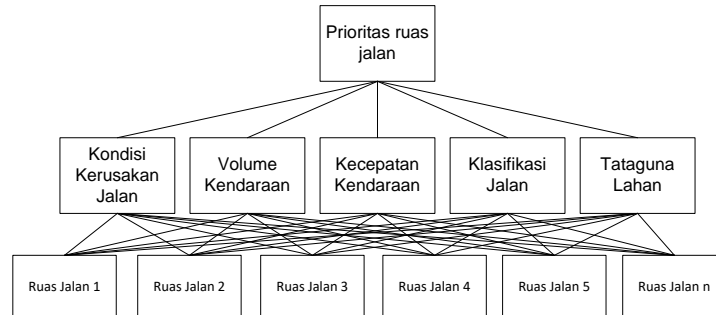
Fig. 3. Struktur Hirarki Kriteria dan Alternatif
