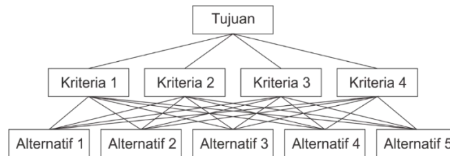
Fig. 1. Struktur Hirarki AHP
